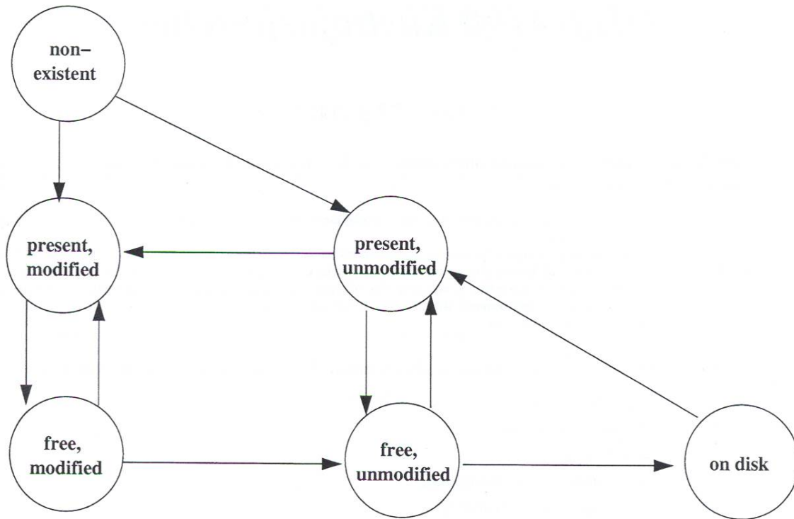
Kuva 1: Muistisivun tilamalli
