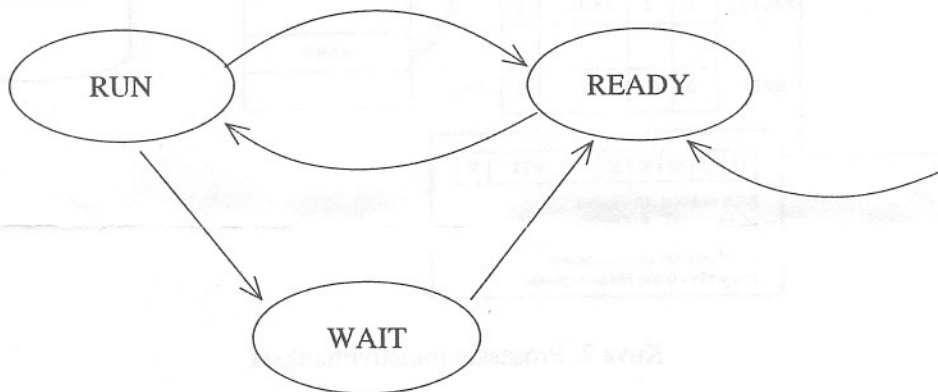
Kuva 1: Sääikeen tilamalli
